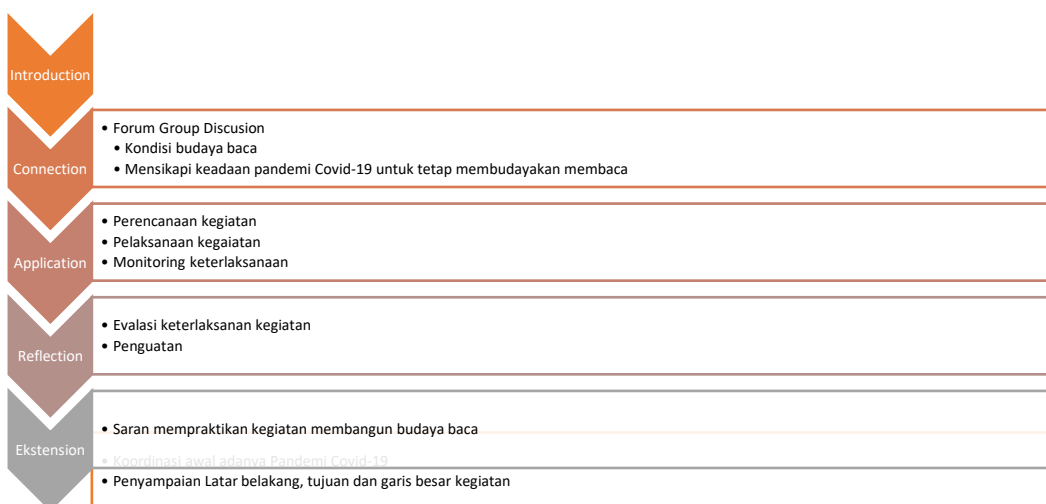
Gambar 1. Metodologi Penelitian
