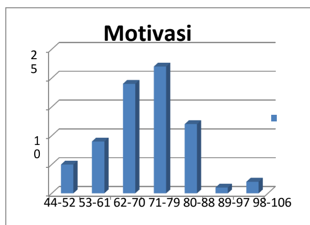
Gambar 2 Histogram Distribusi Frekuensi Data Angket Tentang Motivasi Belajar Pada Mata Pelajaran PPKn
