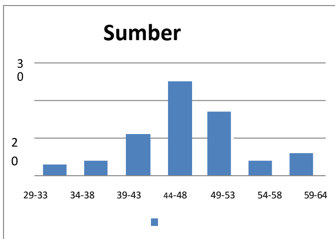
Gambar 1 Histogram Distribusi Frekuensi Kumulatif Data Angket Sumber Belajar
